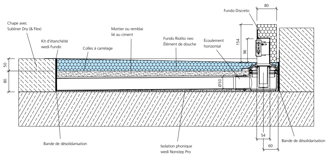
Fundo Discreto, écoulement mural, DN 40, pose sur chape
