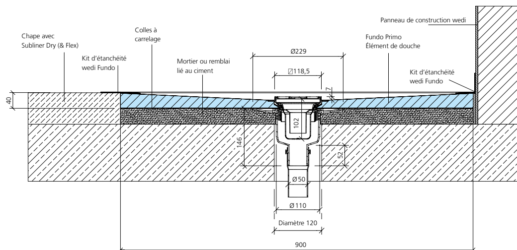
Écoulement en un point wedi Fundo vertical, DN 50, pose sur chape
