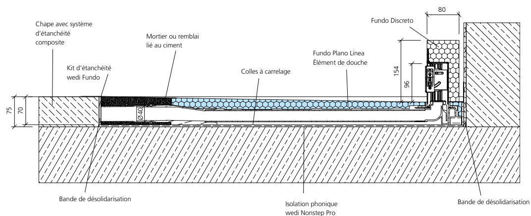
Fundo Discreto, écoulement mural, DN 40, pose sur chape
