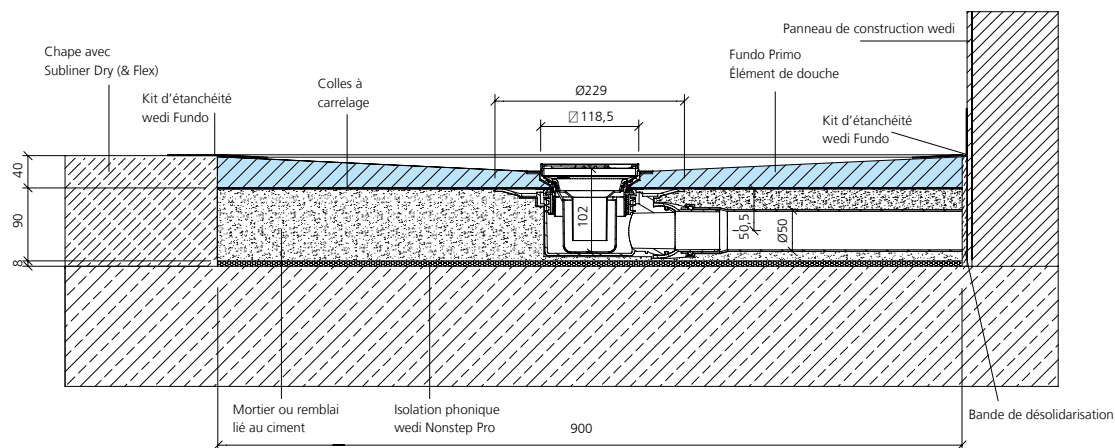
Écoulement en un point wedi Fundo horizontal, DN 50, pose sur chape
