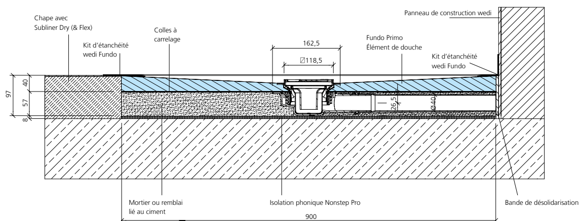
Écoulement en un point wedi Fundo Mini Max, DN 40, pose sur chape
